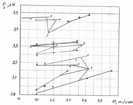
Şəkil 2. İşçi orqanların dartı müqavimətinin ( P_d ) aqreqatın sürətindən ( V ) asılılığı. 1 –qövsvari yumşaldıcı; 2 –kəsmə bucağı dəyişə bilən yastıqası; 3 –ox pəncəli yumşaldıcı.
