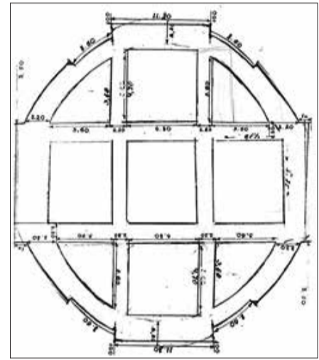
Qüllə formalı binanın sxematik planı
