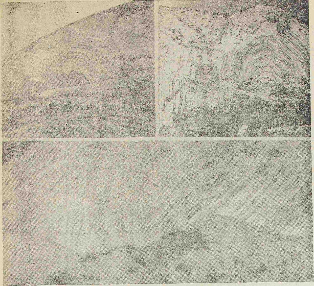
Шәкил 1. Лайларын тәбии гырышыглыгы (фото Н. Гагвердијевиндир) јухарыда (солдан-саға): Кәднесу чајынын сағ саһили; Тудар чајынын сағ саһили; ашағыда: Әнкихәран кәднинин јахынлығында.
