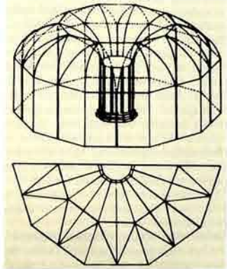
Sərdabə dirayinin konstruksiyası.
