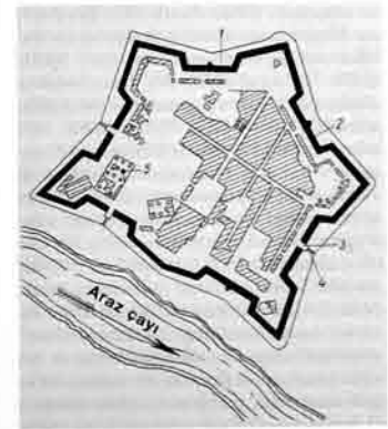
Abbasabad qalasının planı: 1. Kəndək, 2. Qala divarı, 3. Darvaza, 4. Körpü, 5. Bulac
