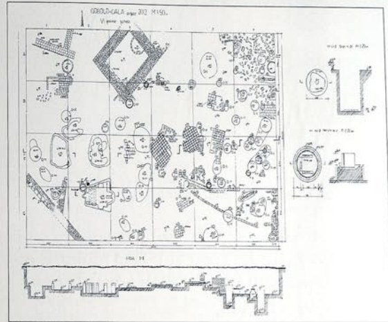
IV qazıntı sahəsinin ümumi planı General plan of the 4th excavation site
