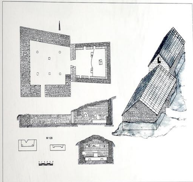
Kilseli Təpə abidəsinin planı (tərtibatçılar: Məhəmməd Əhmədov, Natiq Əlişov) Plan of the Kilseli Tepe monument (drawn up by: Mahammad Ahmadvov, Natig Alishov)
