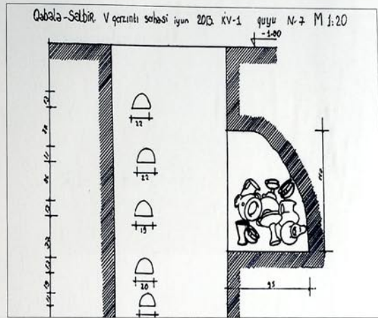
7N-li quyruğu və Antik qəbirin qrafik görünüşü Pit No. 7 and the graphical view of the Ancient grave
