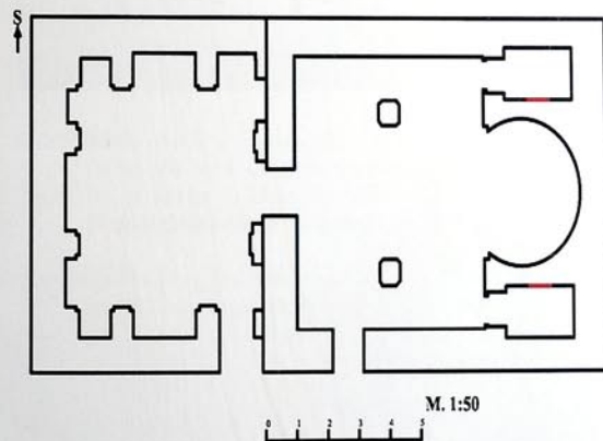
Qarabulaq kilsə-monastırının nartekslə birlikdə planı (tərtibatçı: Natiq Alishov) Plan of the narthex together with the Garabulag church-monastery (drawn up by: Natiq Alishov)
