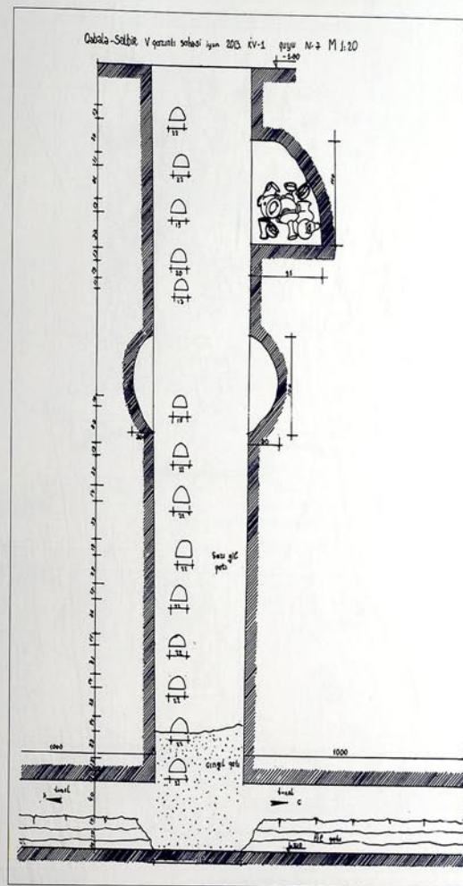
V qazıntı sahəsi, KV1-də aşkarlanmış 7N-li quyunun kəsiyi The 5th excavation site, section of the pit No. 7 detected at the S1
