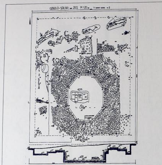
V qazıntı sahəsi, KV2, qazıntının ümumi planı The 5th excavation site, S2, general plan of the excavation
